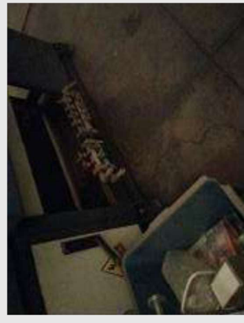
INJETORA HORIZONTAL MARCA HIMACO MOD RAPID 1800-825 LH NS 333271 ANO 1999 | Item: 14 |
